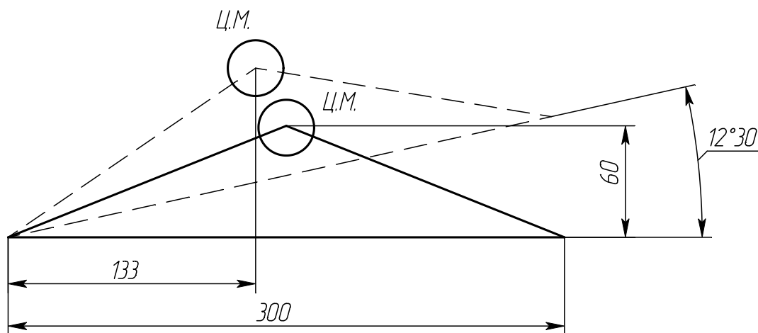
Рисунок 1- Схема устойчивости электронасоса типа 1КМЛ 65-160.
